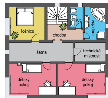
Půdorys rodinného domu BLUES
