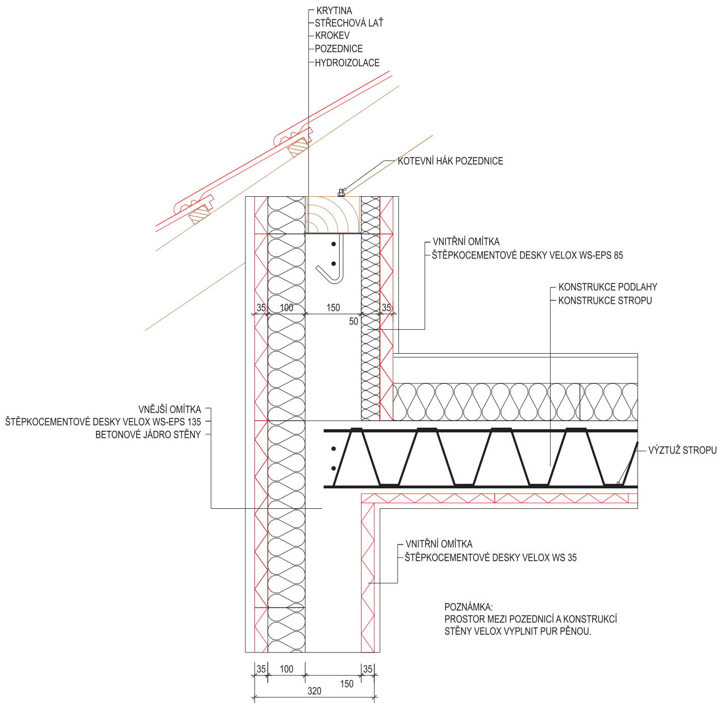
KONSTRUKCE STĚNY VELOX UL 32
