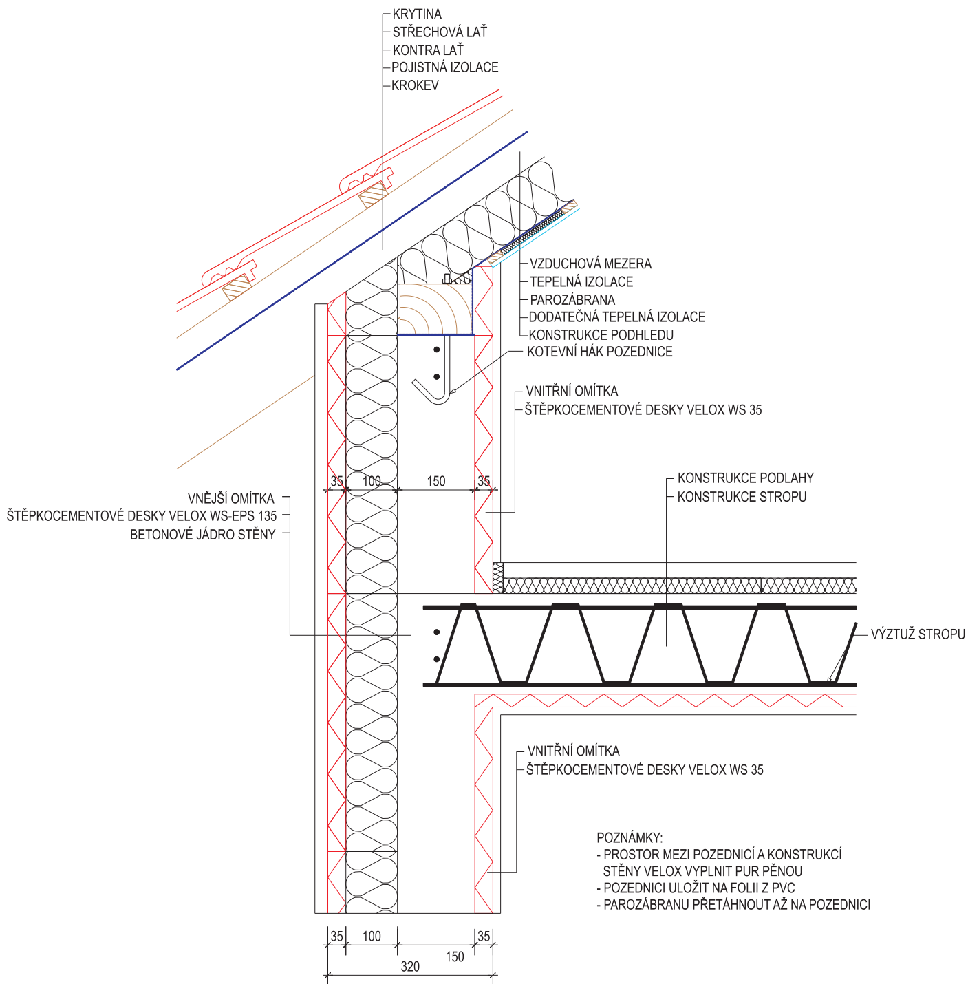
KONSTRUKCE STĚNY VELOX UL 32
