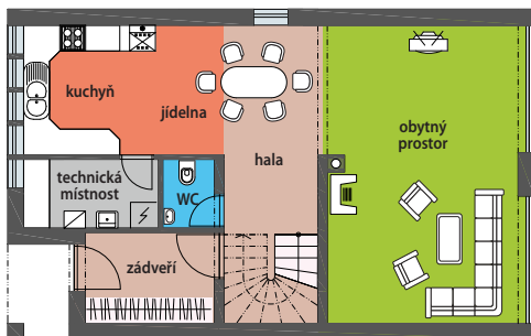
↓ Půdorysy rodinného domu OSIRIS
